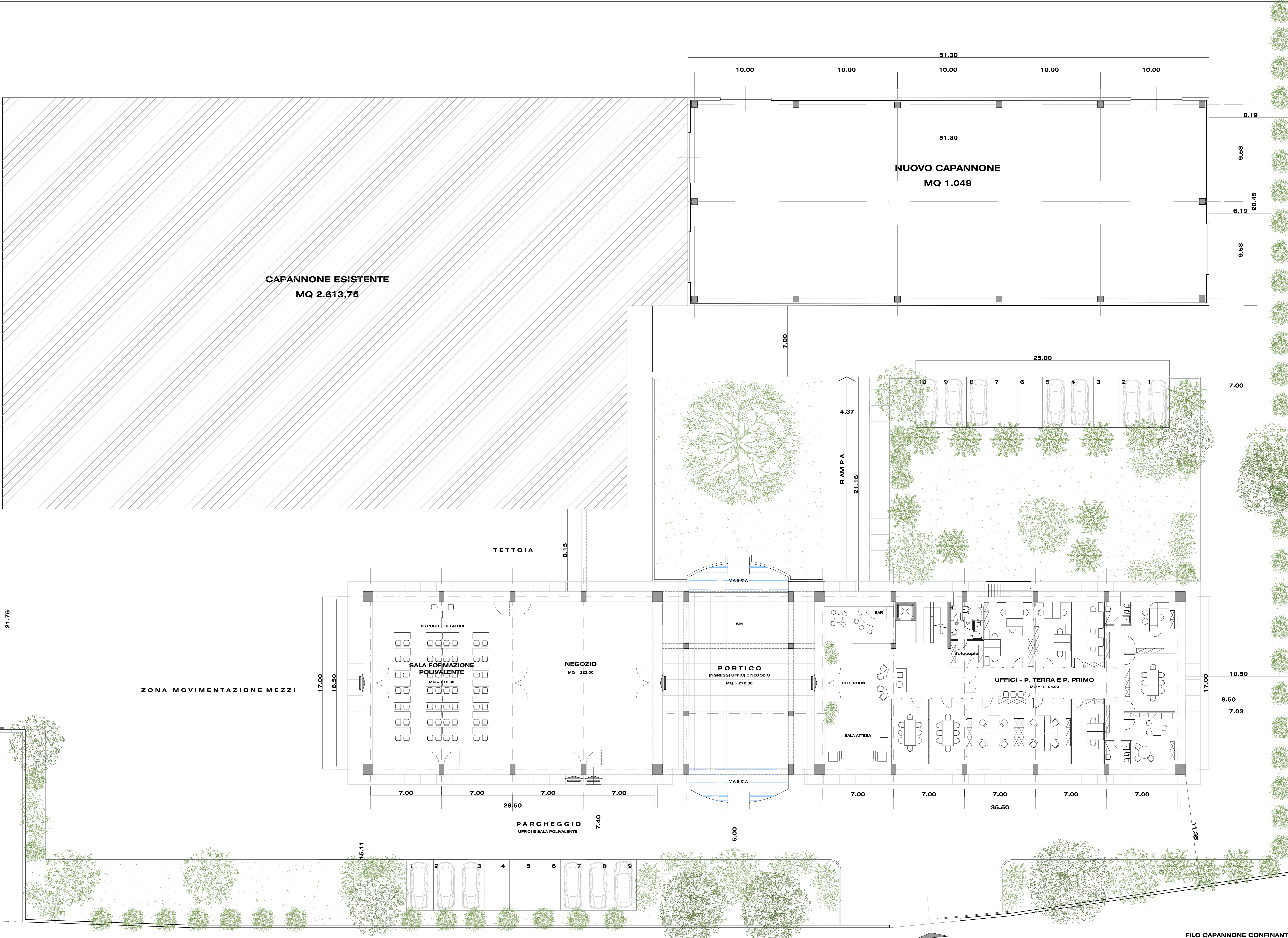
PIANTA PIANO TERRA
